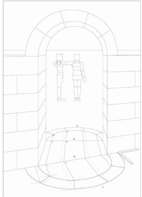
Figura 16. Trazado de las testas del Arco viaje por testa.
