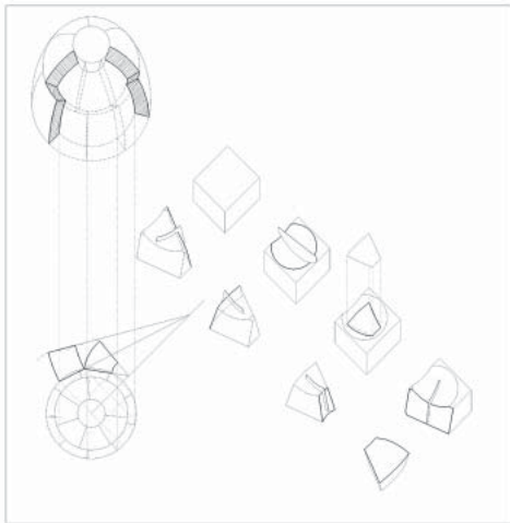
Figura 41. Esquema de trazado y labra de la bóveda esférica.
