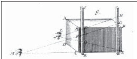
Figura 10. Desalabeo de un sillar. Amedée-Louis Frézier, Traité de stéréotomie , 1737.
